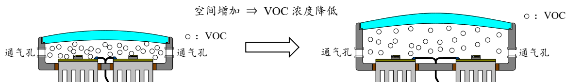
图 8. 对策例 (加大灯具容积)
