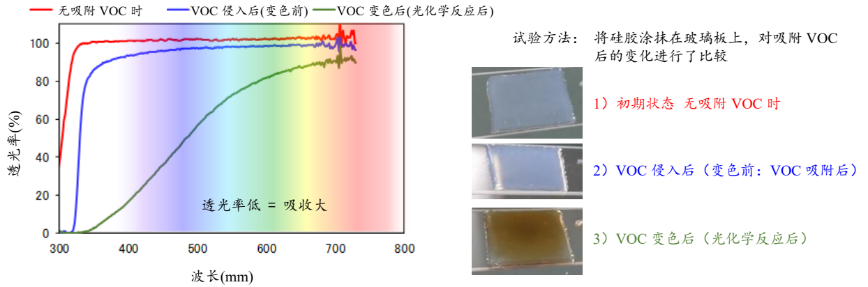
图 5. VOC 的吸附、变色导致的透光率变化
