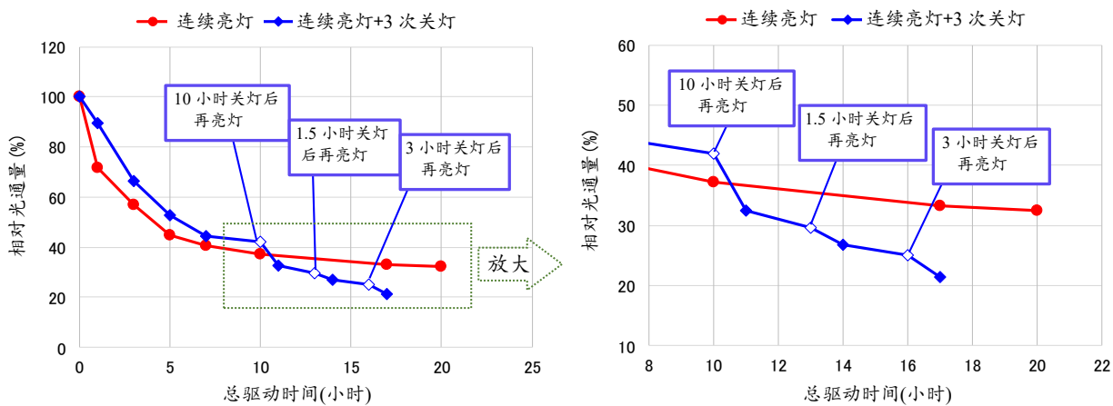
图 14. 连续亮灯和间断亮灯下的光通量下降
