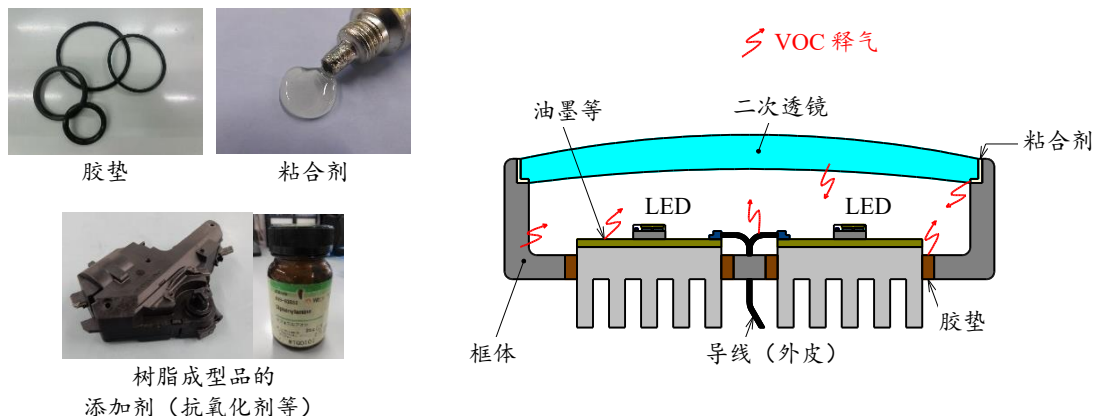
图 2. 可能发生 VOC 的 LED 周边部材例
