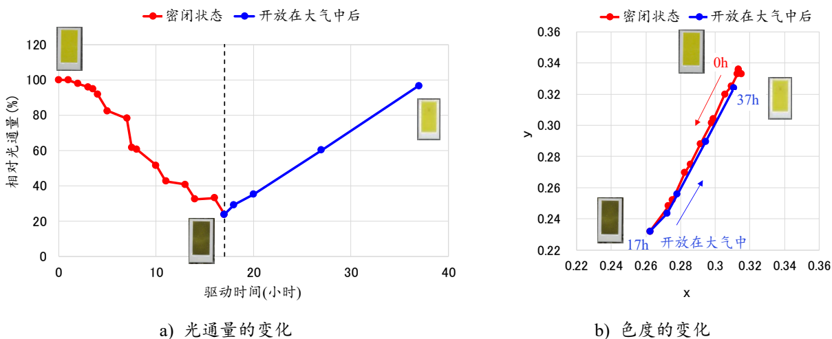
图 12. VOC 变色的发生和减轻 (高浓度 VOC 下的加速验证)
