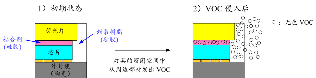
图 4. VOC 侵入时的示意图
