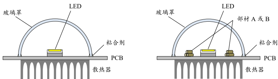
图 10. 试验方法例（左：无试验部材的比较用、右：有试验部材）
