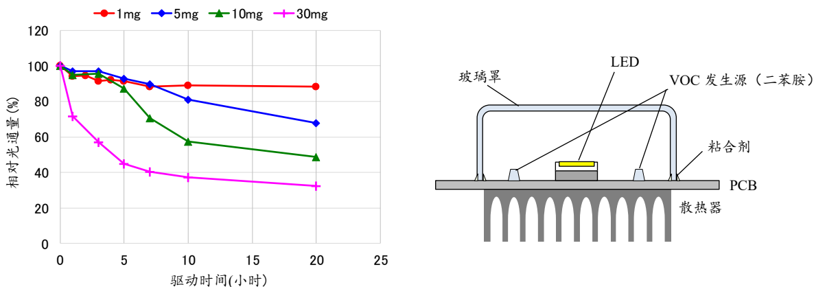
图 13. 发生源（二苯胺）浓度 vs.光通量下降（密闭状态下）
