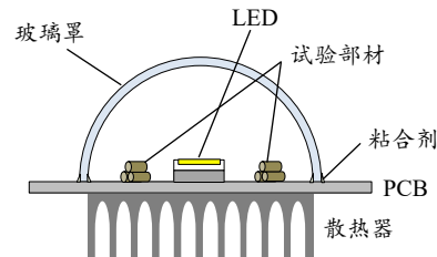
图 9. VOC 变色确认试验例
