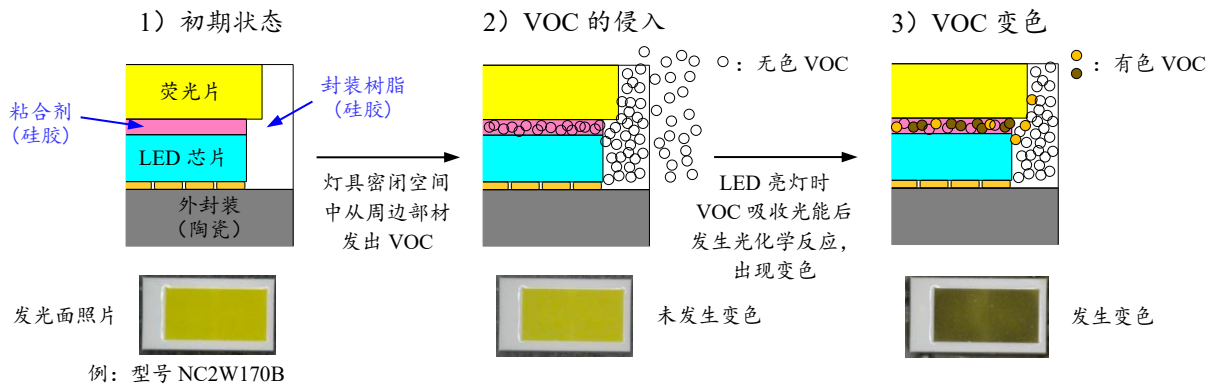
图 6. VOC 变色示意图
