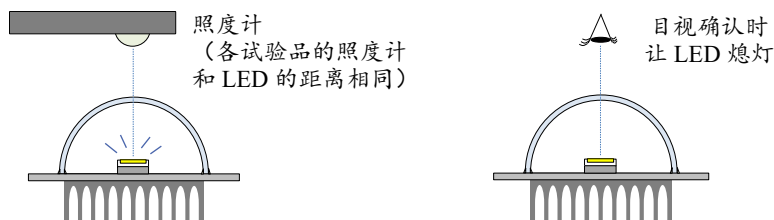
图 11. 光强度和变色的确认
