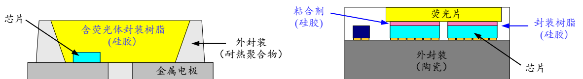
图 3. 使用硅胶的 LED 结构图 (例)
