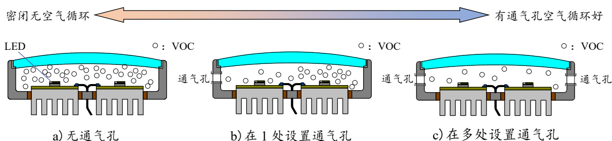
图 7. 对策例 (通气孔的设置)
